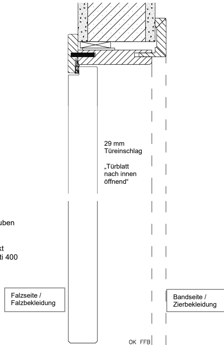
Abb.: Vertikalschnitt
