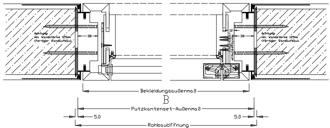
Abb.: Element DIN R
